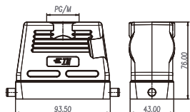
高结构
