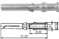
插孔 10A
