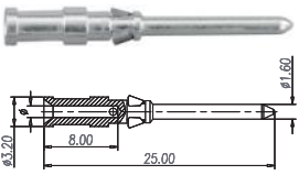
插针 10A
