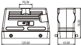
高结构
