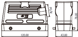
高结构
