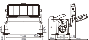
带保护盖
