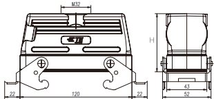
低结构
