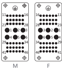
接插针排序
