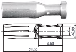
插孔 40A
