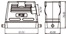
高结构
