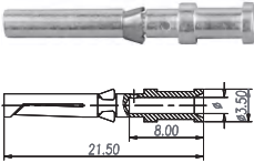
插孔 10A
