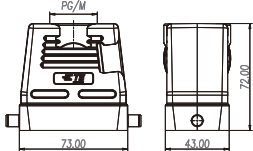
高结构
