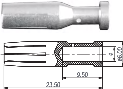
插孔 40A
