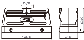
低结构
