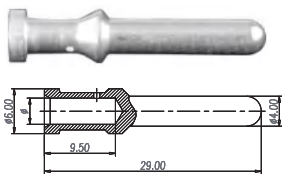
插孔 40A
