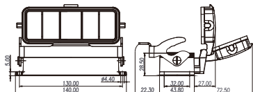
带保护盖
