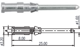
插针 10A
